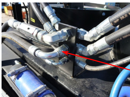
Рис 2: Заглушите шланг (Volvo)
