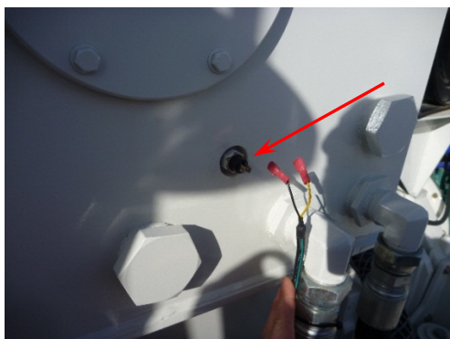
Рис 4: Датчик температуры масла
